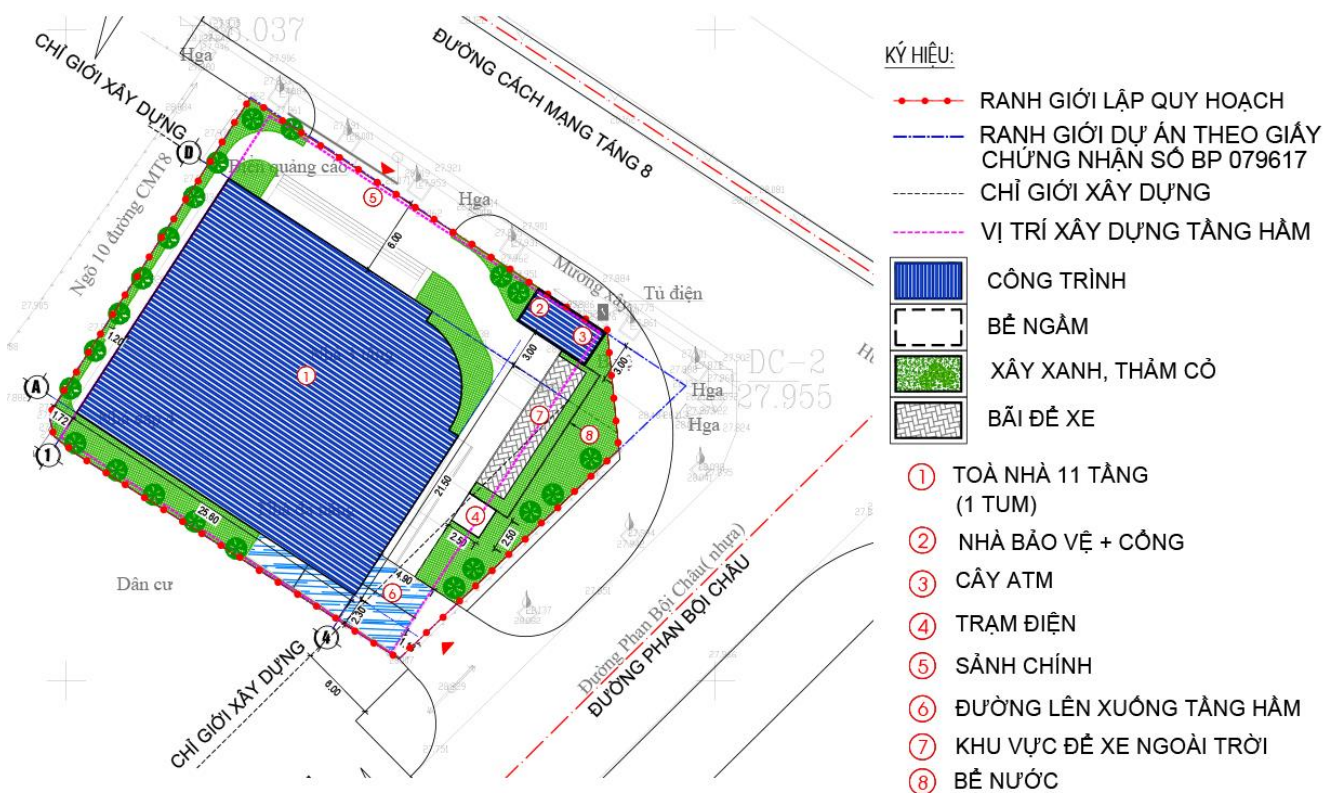
Sơ đồ quy hoạch tổng mặt bằng
